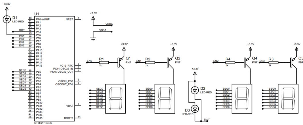
Hình 7: Simulation schematic in Proteus
