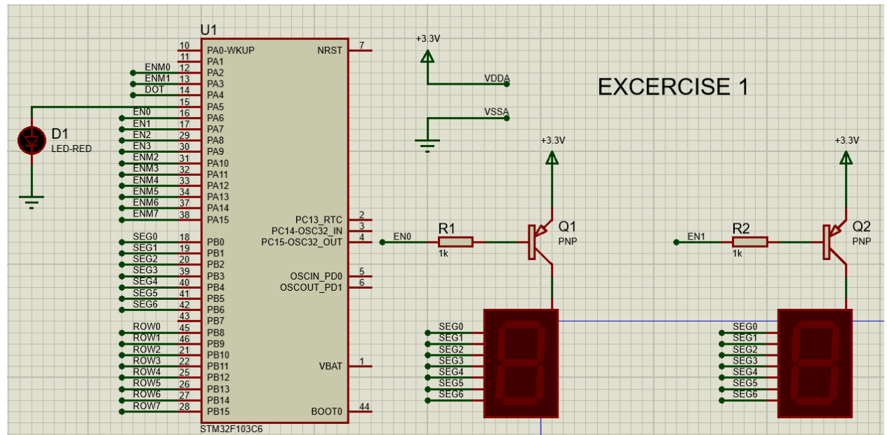
Hình 6: Schematic from Proteus
