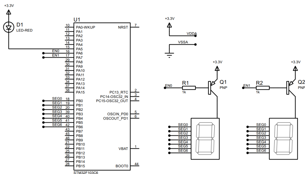
Hình 5: Simulation schematic in Proteus
