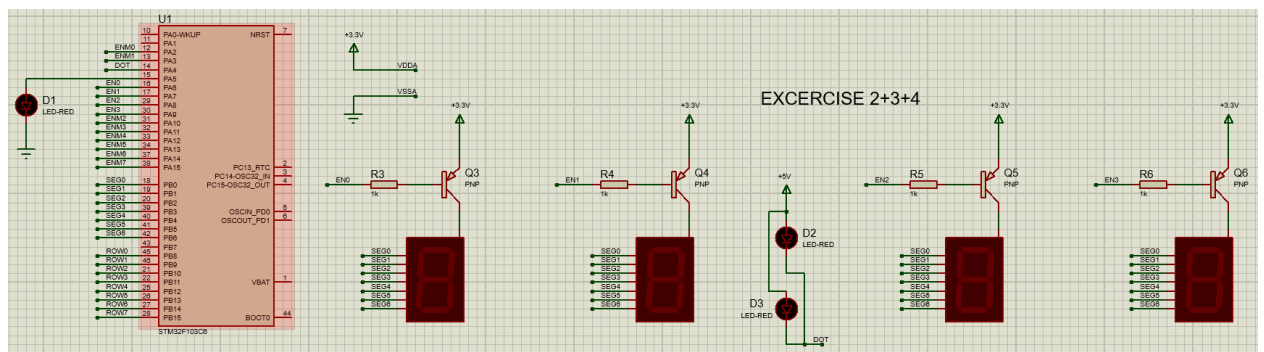
Hình 8: Schematic from Proteus
